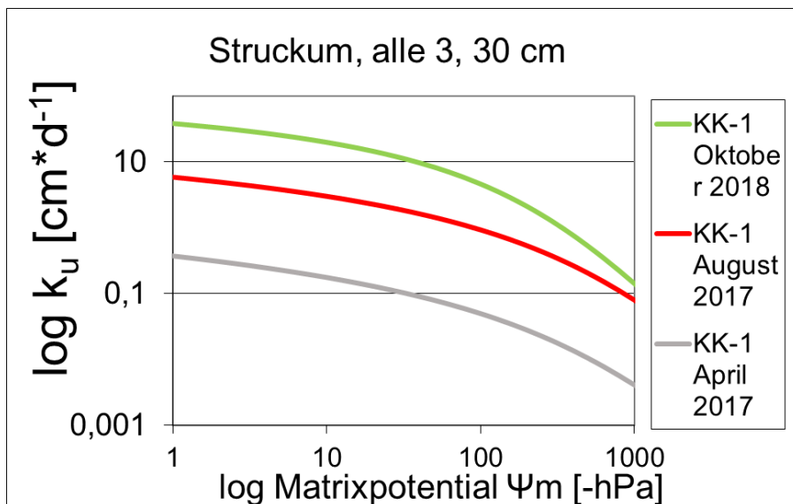
Abbildung 61 Ungesättigte Wasserleitfähigkeit (in \text{cm} \cdot \text{d} ) am Standort Struckum in 30 cm Tiefe für die Variante KK-1 für alle 3 Probenahmen 7, 12 und 26 Monate nach Kalkung, n = 4 .
