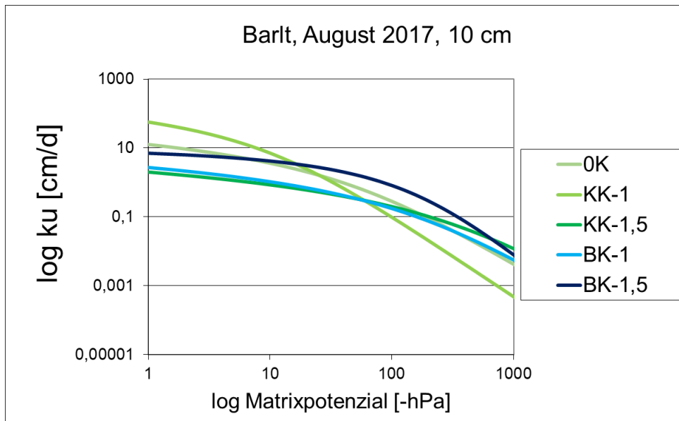
Abbildung 35 Ungesättigte Wasserleitfähigkeit (in \text{cm} \cdot \text{d} ) am Standort Barlt in 10 cm Tiefe, 12 Monate nach Kalkung, n = 4 .
