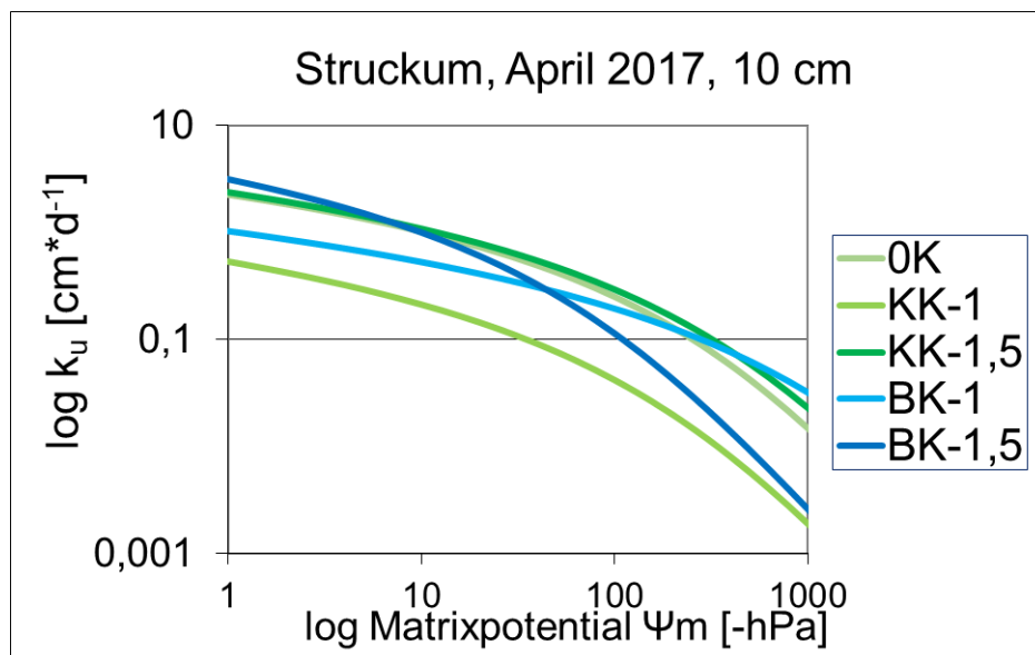
Abbildung 50 Ungesättigte Wasserleitfähigkeit (in \text{cm} \cdot \text{d} ) am Standort Struckum in 10 cm Tiefe, 7 Monate nach Kalkung, n = 4 .
