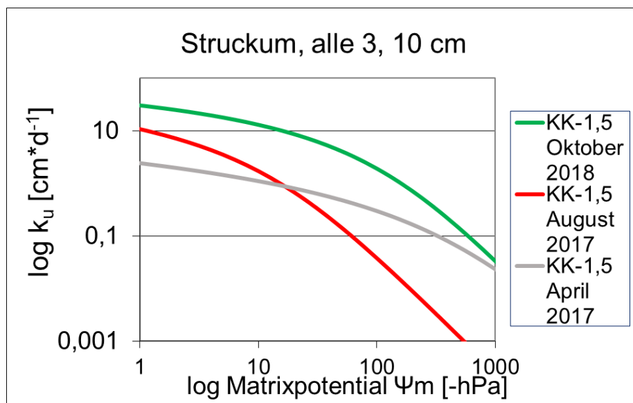
Abbildung 54 Ungesättigte Wasserleitfähigkeit (in \text{cm} \cdot \text{d} ) am Standort Struckum in 10 cm Tiefe für die Variante KK-1,5; für alle 3 Probenahmen 7, 12 und 26 Monate nach Kalkung, n = 4 .
