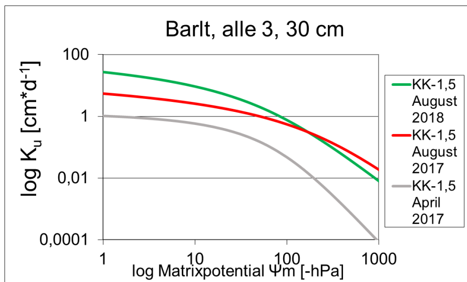
Abbildung 47 Ungesättigte Wasserleitfähigkeit (in \text{cm} \cdot \text{d} ) am Standort Barlt in 30 cm Tiefe für die Variante KK-1,5 für alle 3 Probenahmen 7, 12 und 24 Monate nach Kalkung, n = 4 .
