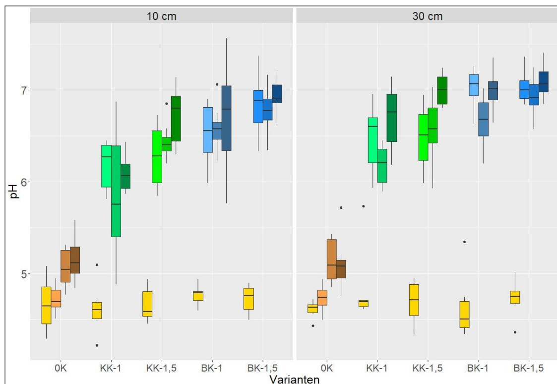
Abbildung 7 pH Werte (in CaCl 2 ) für den Standort Struckum, für 4 verschiedene Zeitpunkte (vor Versuchsanlage, 7, 12 und 26 Monate nach Kalkung); die goldenen Boxplots stellen den Zeitpunkt vor Ausbringen des Kalkes dar. Die drei dunkler werdenden Boxplots pro Variante stellen die drei Probenahmen dar. Die Varianten sind: OK = Nullkalk Referenz, KK-1 = Kohlensaurer Kalk in der einfachen Menge nach VDLUFA Empfehlung für den jeweiligen Standort, KK-1,5 = Kohlensaurer Kalk in der anderthalbfachen Menge nach VDLUFA Empfehlung für den jeweiligen Standort, BK-1 = Brantkalk in der einfachen Menge nach VDLUFA Empfehlung für den jeweiligen Standort, BK-1,5 = Brantkalk in der anderthalbfachen Menge nach VDLUFA Empfehlung für den jeweiligen Standort n = 4
