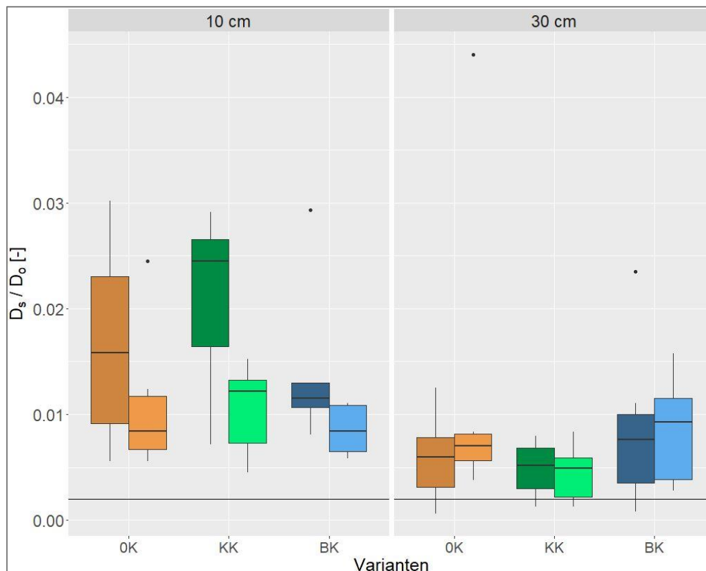
Abbildung 26 Relativer Sauerstoffdiffusionskoeffizient ( D_s/D_o [-]), \Psi_m = -60 hPa, Standort Cunnersdorf an 2 Probenahmen 18 (linker Boxplot) und 23 Monate (rechter Boxplot) nach letzter Kalkung. Die horizontale schwarze Linie steht für einen Wert von 0,002 welcher aus pflanzenbaulicher Sicht ein kritisches Minimum darstellt. Die Varianten sind: OK = Nullkalk Referenz, KK = Kohlensäurer Kalk, BK = Branntkalk. n = 4
