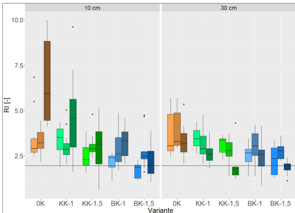
Abbildung 28 Repellency Indices am Standort Struckum (RI, dimensionslos, gemessen bei \Psi_m = -60 hPa) für die Tiefen 10 und 30 cm. Die drei dunkler werdenden Boxplots einer Farbe symbolisieren die drei Probenahmeterminen (7, 12 und 26 Monate nach Kalkung). Die schwarze horizontale Linie verläuft bei einem Wert von 1,95 der nach einigen Literaturquellen als kritischer Grenzwert fungiert, oberhalb dessen Benetzungshemmung auftritt. Die Varianten sind: OK = Nullkalk Referenz, KK-1 = Kohlensaurer Kalk in der einfachen Menge nach VDLUFA Empfehlung für den jeweiligen Standort, KK-1,5 = Kohlensaurer Kalk in der anderthalbfachen Menge nach VDLUFA Empfehlung für den jeweiligen Standort, BK-1 = Branntkalk in der einfachen Menge nach VDLUFA Empfehlung für den jeweiligen Standort, BK-1,5 = Branntkalk in der anderthalbfachen Menge nach VDLUFA Empfehlung für den jeweiligen Standort. n = 12
