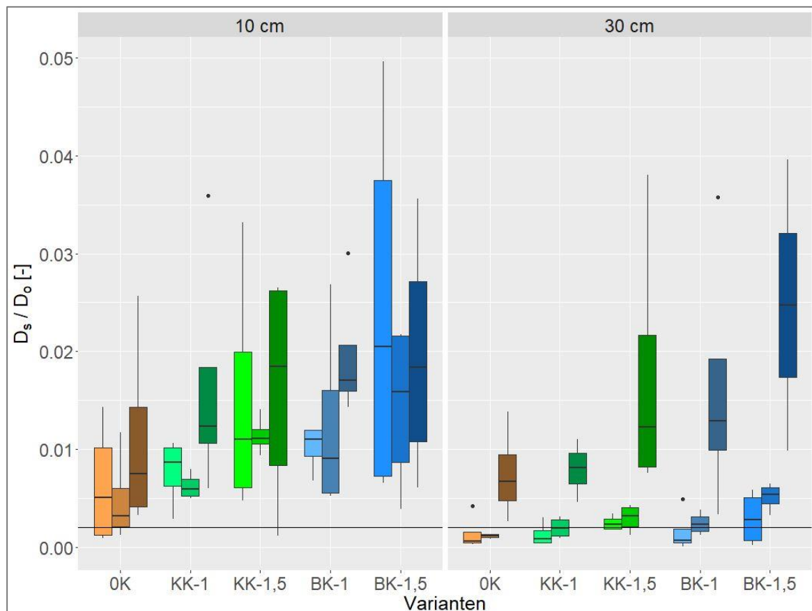
Abbildung 23 Relativer Sauerstoffdiffusionskoeffizient ( D_s/D_o [-]), \Psi_m = -60 hPa, Standort Struckum, 3 Probenahmen (7, 12 und 26 Monate nach Kalkung). Die drei dunkler werdenden Boxplots einer Farbe symbolisieren die drei Probenahmetermine. Die horizontale schwarze Linie steht für einen Wert von 0,002, welcher aus pflanzenbaulicher Sicht ein kritisches Minimum darstellt. Die Varianten sind: OK = Nullkalk Referenz, KK-1 = Kohlensaurer Kalk in der einfachen Menge nach VDLUFA Empfehlung für den jeweiligen Standort, KK-1,5 = Kohlensaurer Kalk in der anderthalbfachen Menge nach VDLUFA Empfehlung für den jeweiligen Standort, BK-1 = Branntkalk in der einfachen Menge nach VDLUFA Empfehlung für den jeweiligen Standort, BK-1,5 = Branntkalk in der anderthalbfachen Menge nach VDLUFA Empfehlung für den jeweiligen Standort. n = 4
