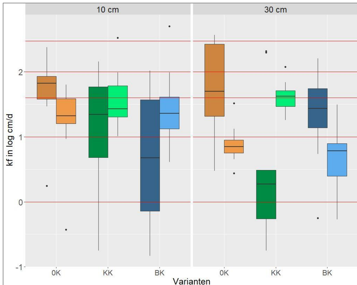
Abbildung 16 Gesättigte Wasserleitfähigkeiten am Standort Cunnersdorf in den Tiefen 10 und 30 cm und für 2 verschiedene Probenahmeterminen 18 Monate (linker Boxplot) und 23 Monate (rechter Boxplot) nach letzter Kalkung). Die roten Linien entsprechen den Grenzwerten der Einstufung nach KA5 (von unten aufsteigend: 1, 10, 40, 100, 300 cm/d). Die Varianten sind: OK = Nullkalk Referenz, KK = Kohlensäurer Kalk, BK = Branntkalk. n = 8
