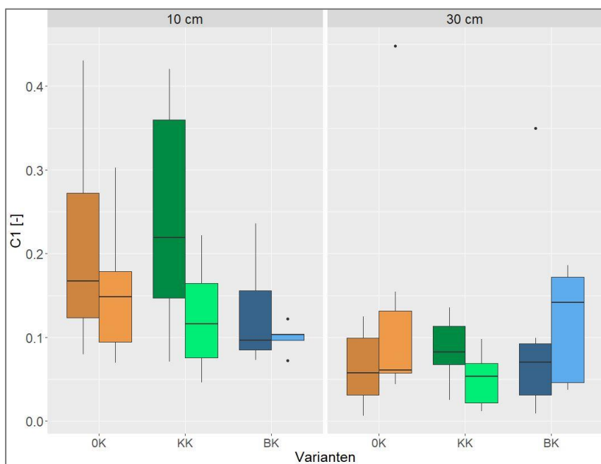
Abbildung 72 C_1 Indices [-] , \Psi_m = -60 hPa, Standort Cunnersdorf an 2 Probenahmen 18 (linker Boxplot) und 23 Monate (rechter Boxplot) nach letzter Kalkung, n = 4 .
