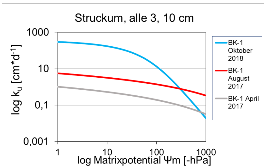
Abbildung 55 Ungesättigte Wasserleitfähigkeit (in \text{cm} \cdot \text{d} ) am Standort Struckum in 10 cm Tiefe für die Variante BK-1, für alle 3 Probenahmen 7, 12 und 26 Monate nach Kalkung, n = 4 .
