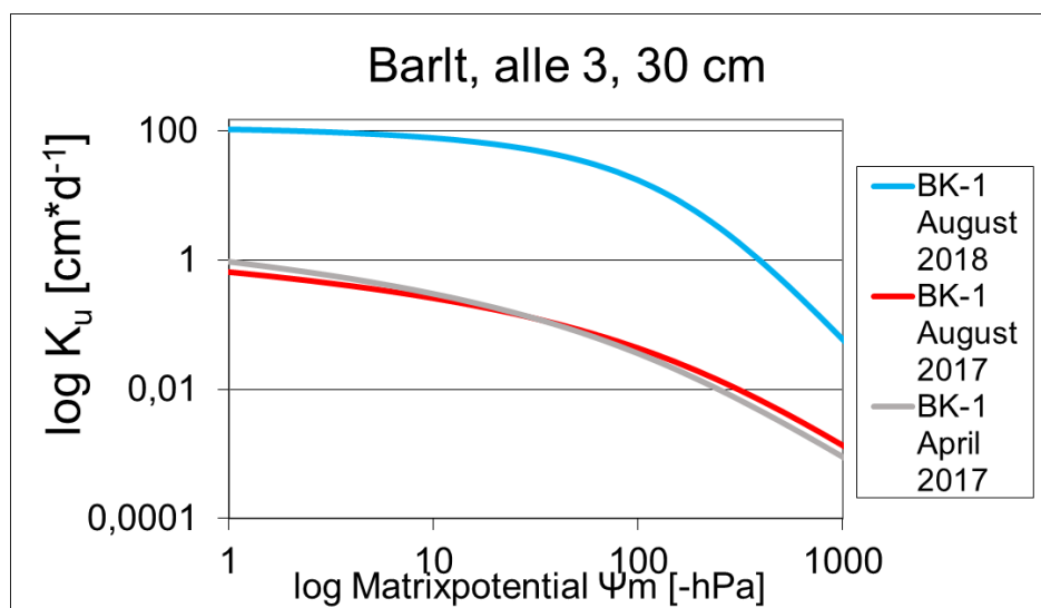
Abbildung 48 Ungesättigte Wasserleitfähigkeit (in \text{cm} \cdot \text{d} ) am Standort Barlt in 30 cm Tiefe für die Variante BK-1 für alle 3 Probenahmen 7, 12 und 24 Monate nach Kalkung, n = 4 .
