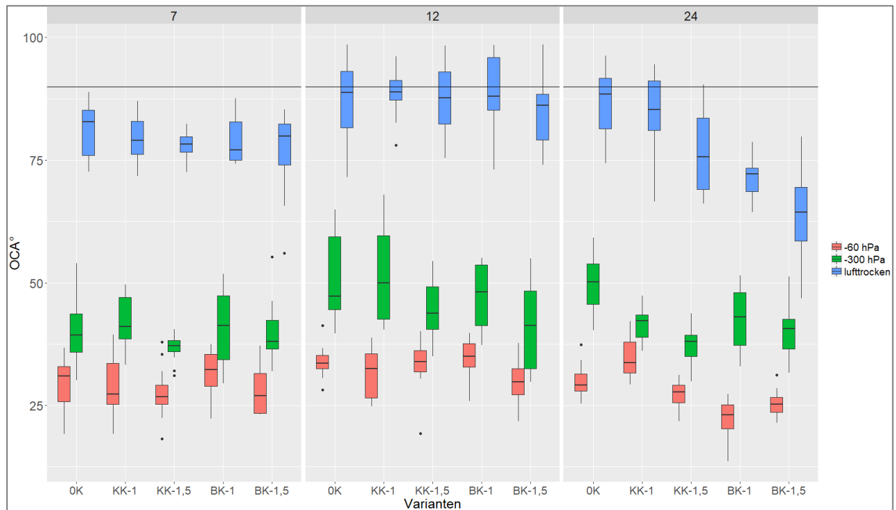
Abbildung 31 Optische Kontaktwinkel am Standort Barlt in 30 cm Tiefe für die drei Probenahmetermine 7, 12 und 24 Monate nach Kalkung, gemessen an 3 unterschiedlichen Entwässerungsstadien (-60 hPa in Rot, -300 hPa in Grün und lufttrocken in Blau). Die schwarze horizontale Linie verläuft bei 90°, oberhalb dessen die Werte als benetzungshemmend gelten (Bachmann et al., 2013). Die Varianten sind: OK = Nullkalk Referenz, KK-1 = Kohlensaurer Kalk in der einfachen Menge nach VDLUFA Empfehlung für den jeweiligen Standort, KK-1,5 = Kohlensaurer Kalk in der anderthalbfachen Menge nach VDLUFA Empfehlung für den jeweiligen Standort, BK-1 = Branntkalk in der einfachen Menge nach VDLUFA Empfehlung für den jeweiligen Standort, BK-1,5 = Branntkalk in der anderthalbfachen Menge nach VDLUFA Empfehlung für den jeweiligen Standort. n = 16
