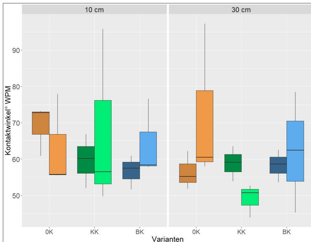
Abbildung 34 Kontaktwinkel nach Wilhelmy-Platten-Methode für den Standort Cunnersdorf. Dargestellt sind die beiden Tiefen 10 und 30 cm, so wie die beiden Probenahmen dargestellt durch den linken Boxplot (18 Monate nach letzter Kalkung) und rechten Boxplot (23 Monate nach letzter Kalkung). Die Varianten sind: OK = Nullkalk Referenz, KK = Kohlensäurer Kalk, BK = Branntkalk. n = 8
