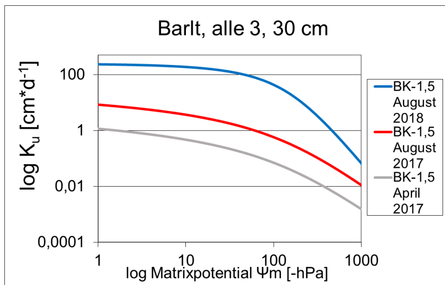
Abbildung 49 Ungesättigte Wasserleitfähigkeit (in \text{cm} \cdot \text{d} ) am Standort Barlt in 30 cm Tiefe für die Variante BK-1,5 für alle 3 Probenahmen 7, 12 und 24 Monate nach Kalkung, n = 4 .
