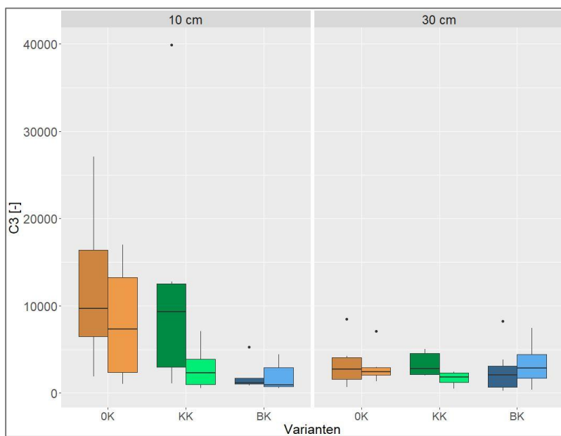
Abbildung 74 C_3 Indices [-], \Psi_m = -60 hPa, Standort Cunnersdorf an 2 Probenahmen 18 (linker Boxplot) und 23 Monate (rechter Boxplot) nach letzter Kalkung, n = 4 .
