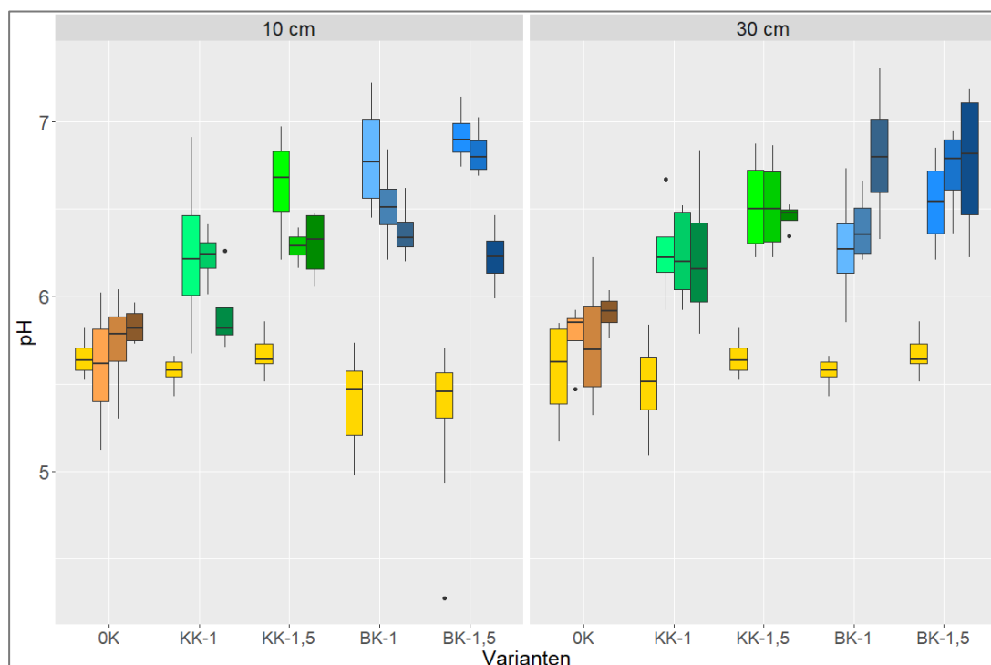
Abbildung 6 pH-Werte (in \text{CaCl}_2 ) für den Standort Barlt, für 4 verschiedene Zeitpunkte (vor Versuchsanlage, 7, 12 und 24 Monate nach Kalkung); die goldenen Boxplots stellen den Zeitpunkt vor Ausbringen des Kalkes dar. Die drei dunkler werdenden Boxplots pro Variante stellen die drei Probenahmen dar. Die Varianten sind: OK = Nullkalk Referenz, KK-1 = Kohlensäurer Kalk in der einfachen Menge nach VDLUFA Empfehlung für den jeweiligen Standort, KK-1,5 = Kohlensäurer Kalk in der anderthalbfachen Menge nach VDLUFA Empfehlung für den jeweiligen Standort, BK-1 =
