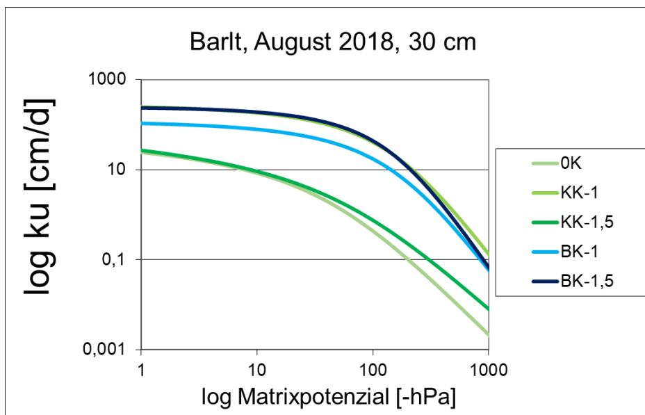
Abbildung 44 Ungesättigte Wasserleitfähigkeit (in \text{cm} \cdot \text{d} ) am Standort Barlt in 30 cm Tiefe, 24 Monate nach Kalkung, n = 4 .
