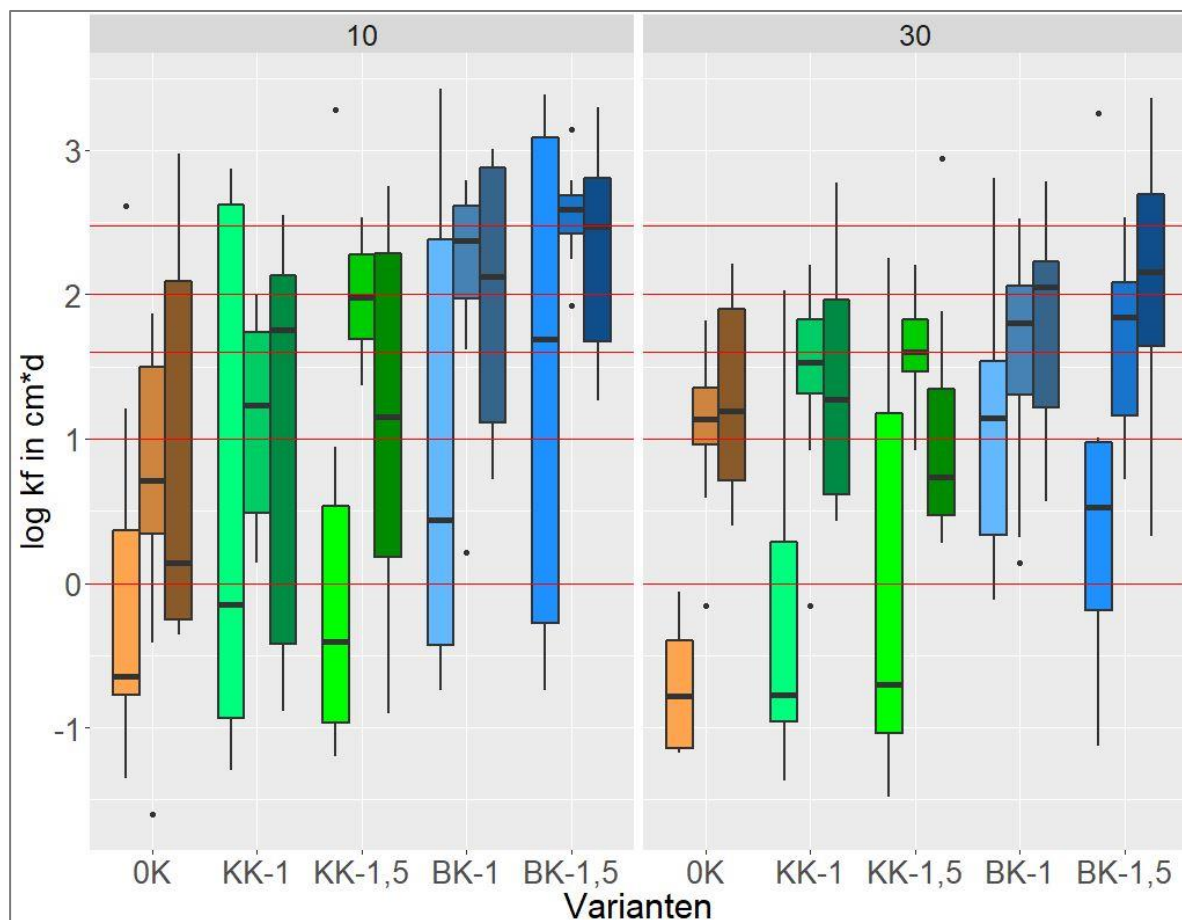
Abbildung 15 Gesättigte Wasserleitfähigkeiten am Standort Struckum in den Tiefen 10 und 30 cm und für drei verschiedene Probenahmeterminen (7, 12 und 26 Monate nach Kalkung), repräsentiert durch die dunkler werdenden Boxplots einer Farbe/Variante. Die roten Linien entsprechen den Grenzwerten der Einstufung nach KA5 (von unten aufsteigend: 1, 10, 40, 100, 300 cm/d). Die Varianten sind: OK = Nullkalk Referenz, KK-1 = Kohlensaurer Kalk in der einfachen Menge nach VDLUFA Empfehlung für den jeweiligen Standort, KK-1,5 = Kohlensaurer Kalk in der anderthalbfachen Menge nach VDLUFA Empfehlung für den jeweiligen Standort, BK-1 = Branntkalk in der einfachen Menge nach VDLUFA Empfehlung für den jeweiligen Standort, BK-1,5 = Branntkalk in der anderthalbfachen Menge nach VDLUFA Empfehlung für den jeweiligen Standort. n = 8
