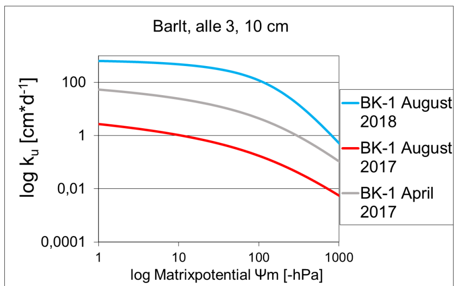
Abbildung 40 Ungesättigte Wasserleitfähigkeit (in \text{cm} \cdot \text{d} ) am Standort Barlt in 10 cm Tiefe für die Variante BK-1 für alle 3 Probenahmen 7, 12 und 24 Monate nach Kalkung, n = 4 .
