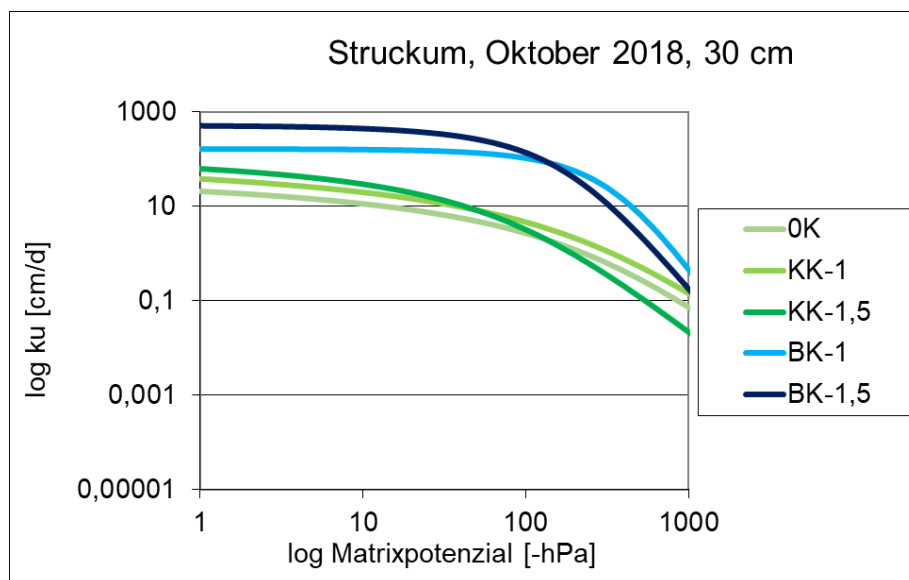
Abbildung 59 Ungesättigte Wasserleitfähigkeit (in \text{cm}^*\text{d} ) am Standort Struckum in 30 cm Tiefe, 26 Monate nach Kalkung, n = 4 .
