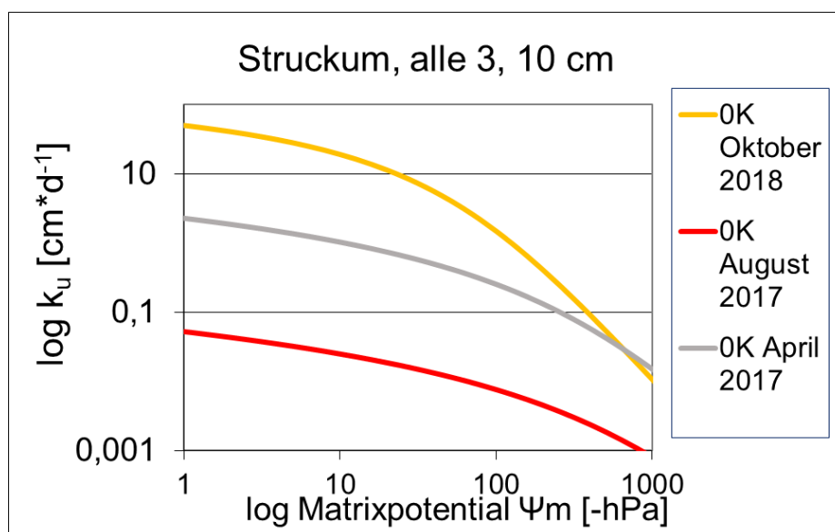
Abbildung 52 Ungesättigte Wasserleitfähigkeit (in \text{cm} \cdot \text{d}^{-1} ) am Standort Struckum in 10 cm Tiefe für die Variante 0K (Nullkalk Referenz) für alle 3 Probenahmen 7, 12 und 26 Monate nach Kalkung, n = 4 .
