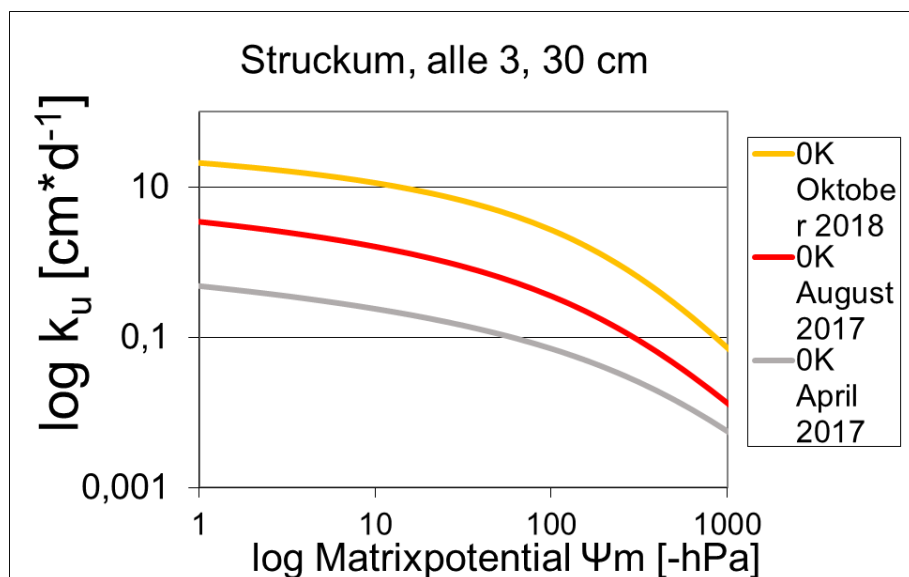
Abbildung 60 Ungesättigte Wasserleitfähigkeit (in \text{cm}^*\text{d} ) am Standort Struckum in 30 cm Tiefe für die Variante 0K (Nullkalk Referenz) für alle 3 Probenahmen 7, 12 und 26 Monate nach Kalkung, n = 4 .
