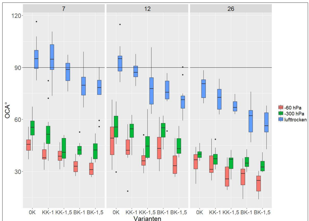
Abbildung 32 Optische Kontaktwinkel am Standort Struckum in 10 cm Tiefe für die drei Probenahmetermine 7, 12 und 26 Monate nach Kalkung, gemessen an 3 unterschiedlichen Entwässerungsstadien (-60 hPa in Rot, -300 hPa in Grün und lufttrocken in Blau). Die schwarze horizontale Linie verläuft bei 90°, oberhalb dessen die Werte als benetzungshemmend gelten (Bachmann et al., 2013). Die Varianten sind: OK = Nullkalk Referenz, KK-1 = Kohlensaurer Kalk in der einfachen Menge nach VDLUFA Empfehlung für den jeweiligen Standort, KK-1,5 = Kohlensaurer Kalk in der anderthalbfachen Menge nach VDLUFA Empfehlung für den jeweiligen Standort, BK-1 = Branntkalk in der einfachen Menge nach VDLUFA Empfehlung für den jeweiligen Standort, BK-1,5 = Branntkalk in der anderthalbfachen Menge nach VDLUFA Empfehlung für den jeweiligen Standort. n = 16
