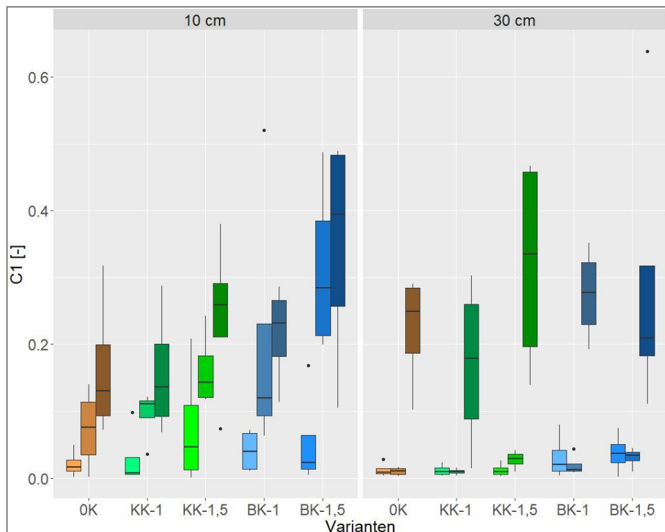
Abbildung 22 C_1 Indices [-], \Psi_m = -60 hPa, Standort Barlt, 3 Probenahmen (7, 12 und 24 Monate nach Kalkung). Die drei dunkler werdenden Boxplots einer Farbe symbolisieren die drei Probenahmeterminen; Die Varianten sind: OK = Nullkalk Referenz, KK-1 = Kohlensaurer Kalk in der einfachen Menge nach VDLUFA Empfehlung für den jeweiligen Standort, KK-1,5 = Kohlensaurer Kalk in der anderthalbfachen Menge nach VDLUFA Empfehlung für den jeweiligen Standort, BK-1 = Brannnkalk in der einfachen Menge nach VDLUFA Empfehlung für den jeweiligen Standort, BK-1,5 = Brannnkalk in der anderthalbfachen Menge nach VDLUFA Empfehlung für den jeweiligen Standort. n=4 .
