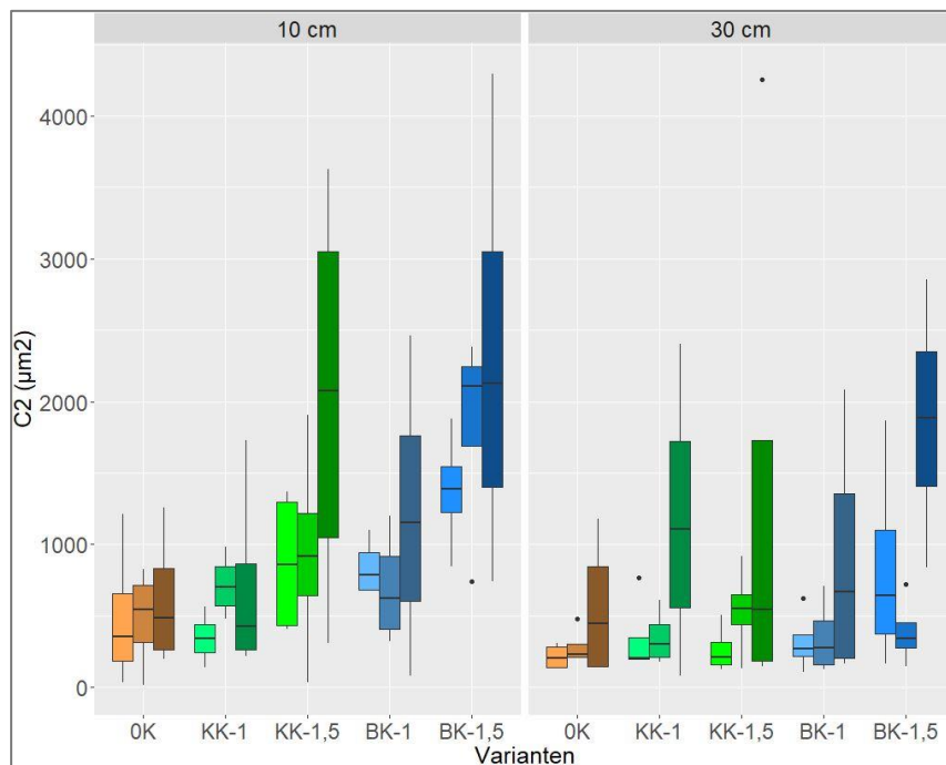
Abbildung 65 C 2 Indices [-], \Psi_m = -60 hPa, Standort Barlt, 3 Probenahmen (7, 12 und 24 Monate nach Kalkung). Die drei dunkler werdenden Boxplots einer Farbe symbolisieren die drei Probenahmeterminen; n= 4.
