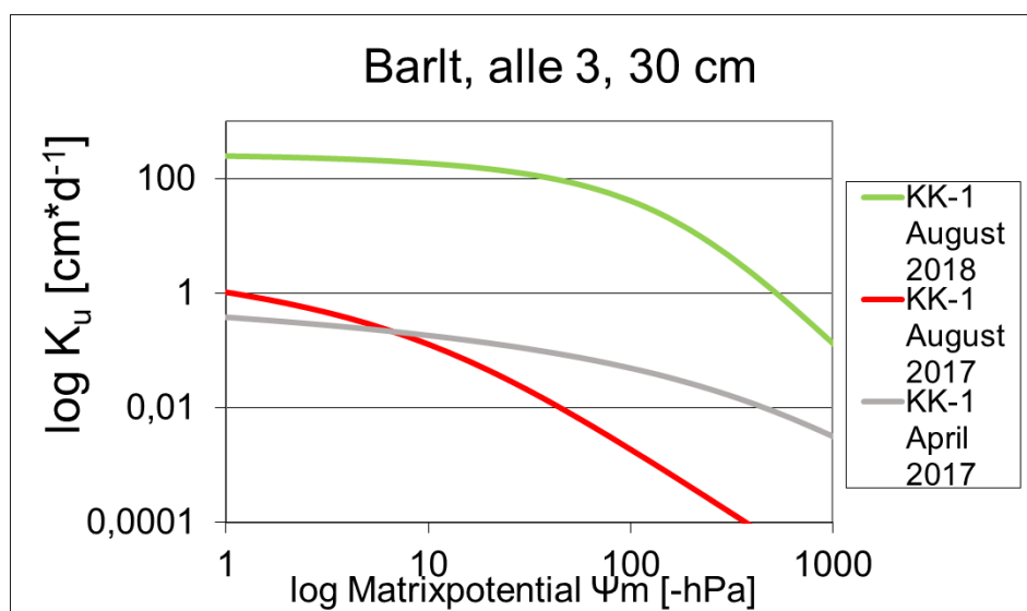
Abbildung 46 Ungesättigte Wasserleitfähigkeit (in \text{cm} \cdot \text{d} ) am Standort Barlt in 30 cm Tiefe für die Variante KK-1 für alle 3 Probenahmen 7, 12 und 24 Monate nach Kalkung, n = 4 .
