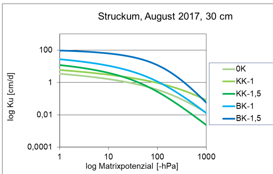
Abbildung 58 Ungesättigte Wasserleitfähigkeit (in \text{cm} \cdot \text{d} ) am Standort Struckum in 30 cm Tiefe, 12 Monate nach Kalkung, n = 4 .
