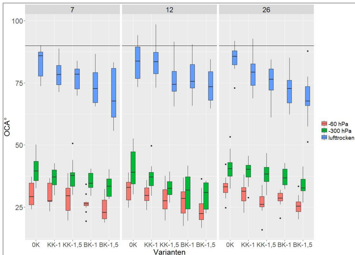
Abbildung 33 Optische Kontaktwinkel am Standort Struckum in 30 cm Tiefe für die drei Probenahmeterminen 7, 12 und 26 Monate nach Kalkung, gemessen an 3 unterschiedlichen Entwässerungsstadien (-60 hPa in Rot, -300 hPa in Grün und lufttrocken in Blau). Die schwarze horizontale Linie verläuft bei 90°, oberhalb dessen die Werte als benetzungshemmend gelten (Bachmann et al., 2013). Die Varianten sind: OK = Nullkalk Referenz, KK-1 = Kohlensäurer Kalk in der einfachen Menge nach VDLUFA Empfehlung für den jeweiligen Standort, KK-1,5 = Kohlensäurer Kalk in der anderthalbfachen Menge nach VDLUFA Empfehlung für den jeweiligen Standort, BK-1 = Branntkalk in der
