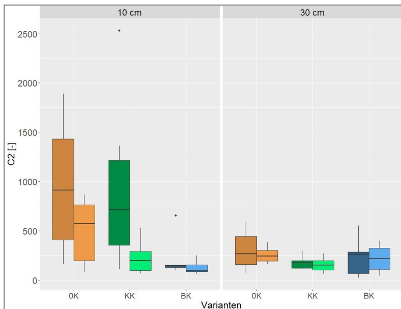
Abbildung 73 C_2 Indices [-], \Psi_m = -60 hPa, Standort Cunnersdorf an 2 Probenahmen 18 (linker Boxplot) und 23 Monate (rechter Boxplot) nach letzter Kalkung, n = 4 .
