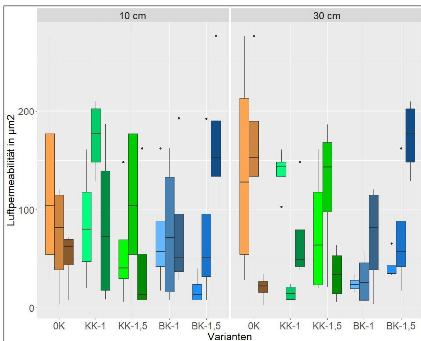
Abbildung 70 Luftpermeabilität (in µm²), \Psi_m = -60 hPa, Standort Struckum, 3 Probenahmen (7, 12 und 26 Monate nach Kalkung). Die drei dunkler werdenden Boxplots einer Farbe symbolisieren die drei Probenahmetermine; n = 4 .
