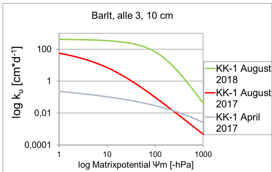
Abbildung 38 Ungesättigte Wasserleitfähigkeit (in \text{cm} \cdot \text{d} ) am Standort Barlt in 10 cm Tiefe für die Variante KK-1 für alle 3 Probenahmen 7, 12 und 24 Monate nach Kalkung, n = 4 .
