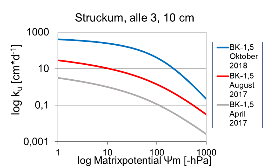
Abbildung 56 Ungesättigte Wasserleitfähigkeit (in \text{cm} \cdot \text{d} ) am Standort Struckum in 10 cm Tiefe für die Variante BK-1,5; für alle 3 Probenahmen 7, 12 und 26 Monate nach Kalkung, n = 4 .
