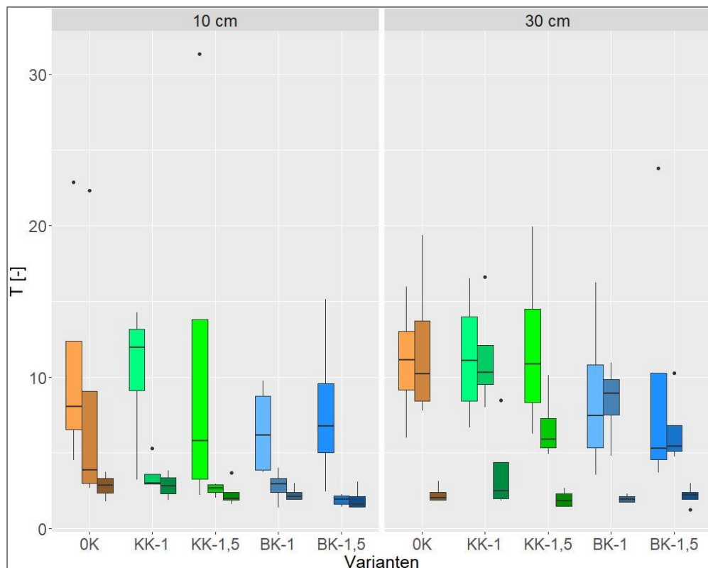
Abbildung 21 Tortuositätsindices ( T [-] ), \Psi_m = -60 hPa, Standort Barlt, 3 Probenahmen (7, 12 und 24 Monate nach Kalkung). Die drei dunkler werdenden Boxplots einer Farbe symbolisieren die drei Probenahmetermine; Die Varianten sind: OK = Nullkalk Referenz, KK-1 = Kohlensaurer Kalk in der einfachen Menge nach VDLUFA Empfehlung für den jeweiligen Standort, KK-1,5 = Kohlensaurer Kalk in der anderthalbfachen Menge nach VDLUFA Empfehlung für den jeweiligen Standort, BK-1 = Branntkalk in der einfachen Menge nach VDLUFA Empfehlung für den jeweiligen Standort, BK-1,5 = Branntkalk in der anderthalbfachen Menge nach VDLUFA Empfehlung für den jeweiligen Standort. n=4 .
