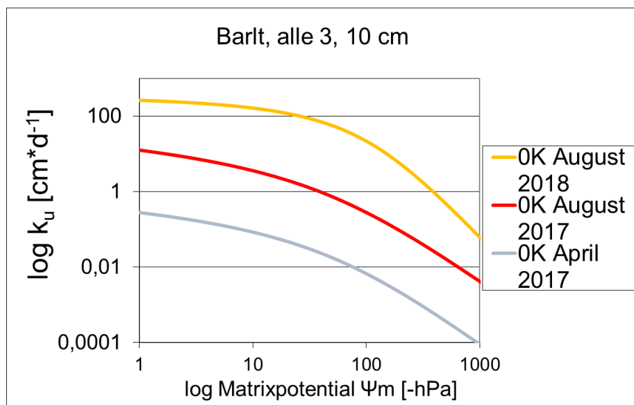
Abbildung 37 Ungesättigte Wasserleitfähigkeit (in \text{cm} \cdot \text{d} ) am Standort Barlt in 10 cm Tiefe für die Variante 0K (Nullkalk Referenz) für alle 3 Probenahmen 7, 12 und 24 Monate nach Kalkung, n = 4 .
