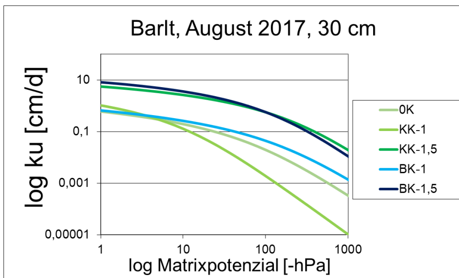
Abbildung 43 Ungesättigte Wasserleitfähigkeit (in \text{cm} \cdot \text{d} ) am Standort Barlt in 30 cm Tiefe, 12 Monate nach Kalkung, n = 4 .
