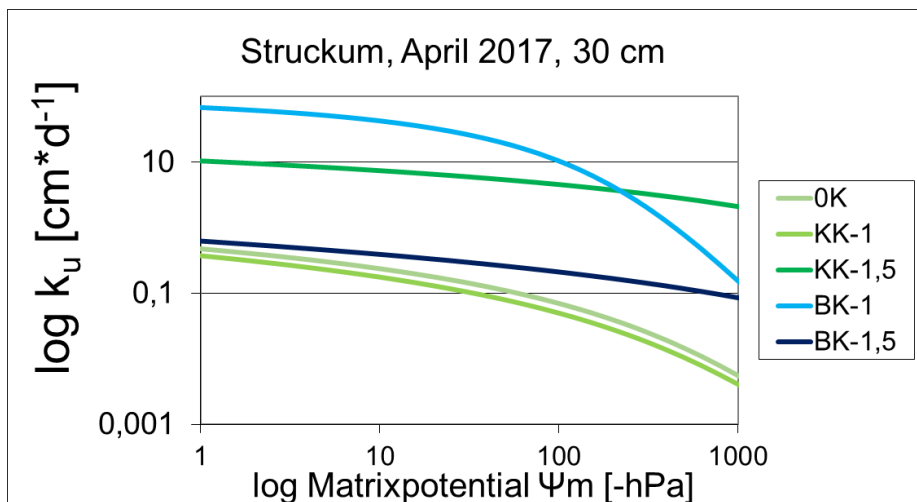
Abbildung 57 Ungesättigte Wasserleitfähigkeit (in \text{cm} \cdot \text{d} ) am Standort Struckum in 30 cm Tiefe, 7 Monate nach Kalkung, n = 4 .
