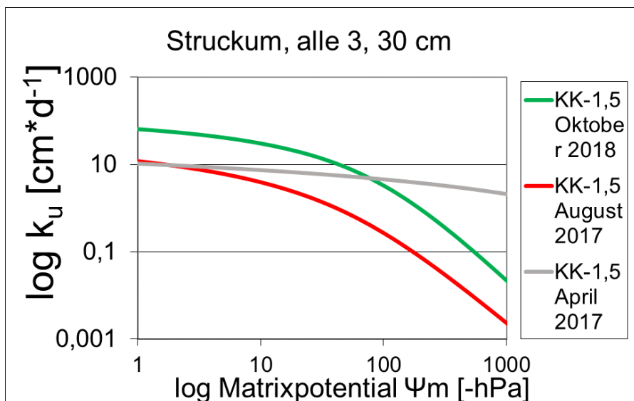
Abbildung 62 Ungesättigte Wasserleitfähigkeit (in \text{cm} \cdot \text{d} ) am Standort Struckum in 30 cm Tiefe für die Variante KK-1,5 für alle 3 Probenahmen 7, 12 und 26 Monate nach Kalkung, n = 4 .
