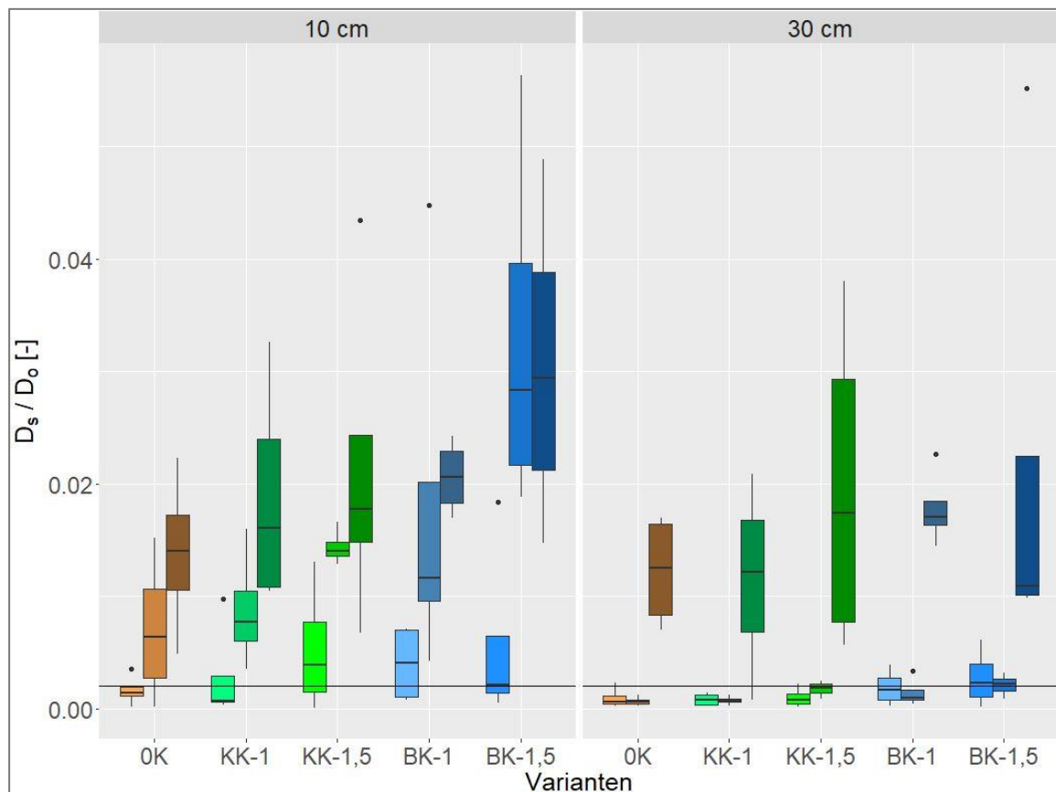
Abbildung 20 Relativer Sauerstoffdiffusionskoeffizient ( D_s/D_o [-] ), \Psi_m = -60 hPa, Standort Barlt, 3 Probenahmen (7, 12 und 24 Monate nach Kalkung). Die drei dunkler werdenden Boxplots einer Farbe symbolisieren die drei Probenahmeterminen. Die horizontale schwarze Linie steht für einen Wert von 0,002 welcher aus pflanzenbaulicher Sicht ein kritisches Minimum darstellt. Die Varianten sind: OK = Nullkalk Referenz, KK-1 = Kohlensaurer Kalk in der einfachen Menge nach VDLUFA Empfehlung für den jeweiligen Standort, KK-1,5 = Kohlensaurer Kalk in der anderthalbfachen Menge nach VDLUFA Empfehlung für den jeweiligen Standort, BK-1 = Branntkalk in der einfachen Menge nach VDLUFA Empfehlung für den jeweiligen Standort, BK-1,5 = Branntkalk in der anderthalbfachen Menge nach VDLUFA Empfehlung für den jeweiligen Standort. n = 4
