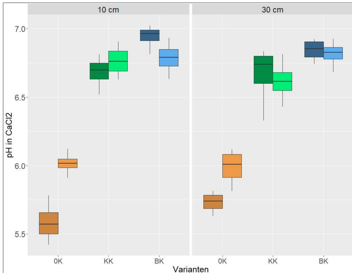
Abbildung 8 pH-Werte (in CaCl 2 ) für den Standort Cunnersdorf, für 2 verschiedene Zeitpunkte (April 2016 linker Teil der Boxplot-Paare, August 2016 rechter Teil der Boxplot-Paare). Die Varianten sind: OK = Nullkalk Referenz, KK = Kohlensäurer Kalk, BK = Branntkalk. n = 4
