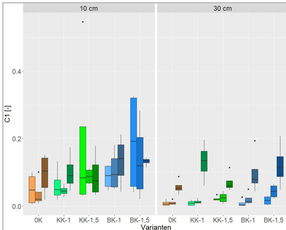
Abbildung 25 C_1 Indices [-], \Psi_m = -60 hPa, Standort Struckum, 3 Probenahmen (7, 12 und 26 Monate nach Kalkung). Die drei dunkler werdenden Boxplots einer Farbe symbolisieren die drei Probenahmetermine; Die Varianten sind: OK = Nullkalk Referenz, KK-1 = Kohlensaurer Kalk in der einfachen Menge nach VDLUFA Empfehlung für den jeweiligen Standort, KK-1,5 = Kohlensaurer Kalk in der anderthalbfachen Menge nach VDLUFA Empfehlung für den jeweiligen Standort, BK-1 = Branntkalk in der einfachen Menge nach VDLUFA Empfehlung für den jeweiligen Standort, BK-1,5 = Branntkalk in der anderthalbfachen Menge nach VDLUFA Empfehlung für den jeweiligen Standort. n=4 .
