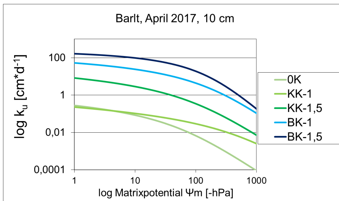
Abbildung 17 Ungesättigte Wasserleitfähigkeit ( k_u in \text{cm} \cdot \text{d} ) für den Standort Barlt in 10 cm Tiefe, 7 Monate nach Kalkung. Die Varianten sind: 0K = Nullkalk Referenz, KK-1 = Kohlensaurer Kalk in der einfachen Menge nach VDLUFA Empfehlung für den jeweiligen Standort, KK-1,5 = Kohlensaurer Kalk in der anderthalbfachen Menge nach VDLUFA Empfehlung für den jeweiligen Standort, BK-1 = Branntkalk in der einfachen Menge nach VDLUFA Empfehlung für den
