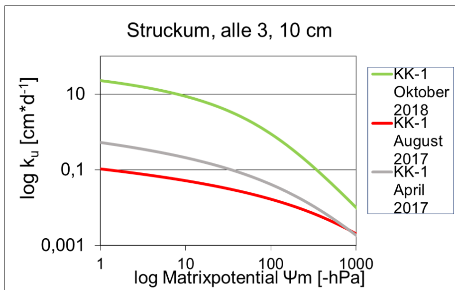
Abbildung 53 Ungesättigte Wasserleitfähigkeit (in \text{cm} \cdot \text{d} ) am Standort Struckum in 10 cm Tiefe für die Variante KK-1, für alle 3 Probenahmen 7, 12 und 26 Monate nach Kalkung, n = 4 .
