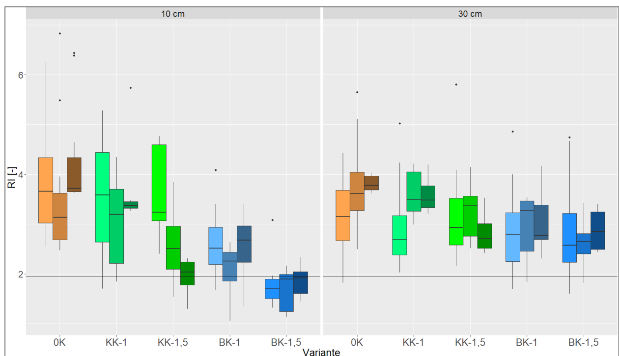
Abbildung 27 Repellency Indices am Standort Barlt (RI, dimensionslos, gemessen bei \Psi_m = -60 hPa) für die Tiefen 10 und 30 cm. Die drei dunkler werdenden Boxplots einer Farbe symbolisieren die drei Probenahmetermine (7, 12 und 24 Monate nach Kalkung). Die schwarze horizontale Linie verläuft bei einem Wert von 1,95 der nach einigen Literaturquellen als kritischer Grenzwert fungiert, oberhalb dessen Benetzungshemmung auftritt. Die Varianten sind: OK = Nullkalk Referenz, KK-1 = Kohlensaurer Kalk in der einfachen Menge nach VDLUFA Empfehlung für den jeweiligen Standort, KK-1,5 = Kohlensaurer Kalk in der anderthalbfachen Menge nach VDLUFA Empfehlung für den jeweiligen Standort, BK-1 = Branntkalk in der einfachen Menge nach VDLUFA Empfehlung für den jeweiligen Standort, BK-1,5 = Branntkalk in der anderthalbfachen Menge nach VDLUFA Empfehlung für den jeweiligen Standort. n = 12
