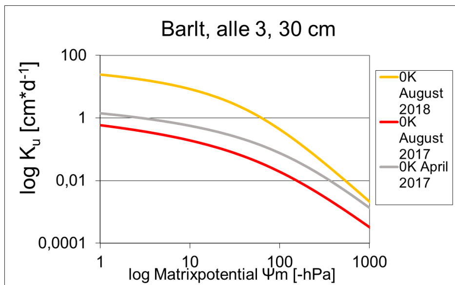
Abbildung 45 Ungesättigte Wasserleitfähigkeit (in \text{cm} \cdot \text{d} ) am Standort Barlt in 30 cm Tiefe für die Variante OK (Nullkalk Referenz) für alle 3 Probenahmen 7, 12 und 24 Monate nach Kalkung, n = 4 .
