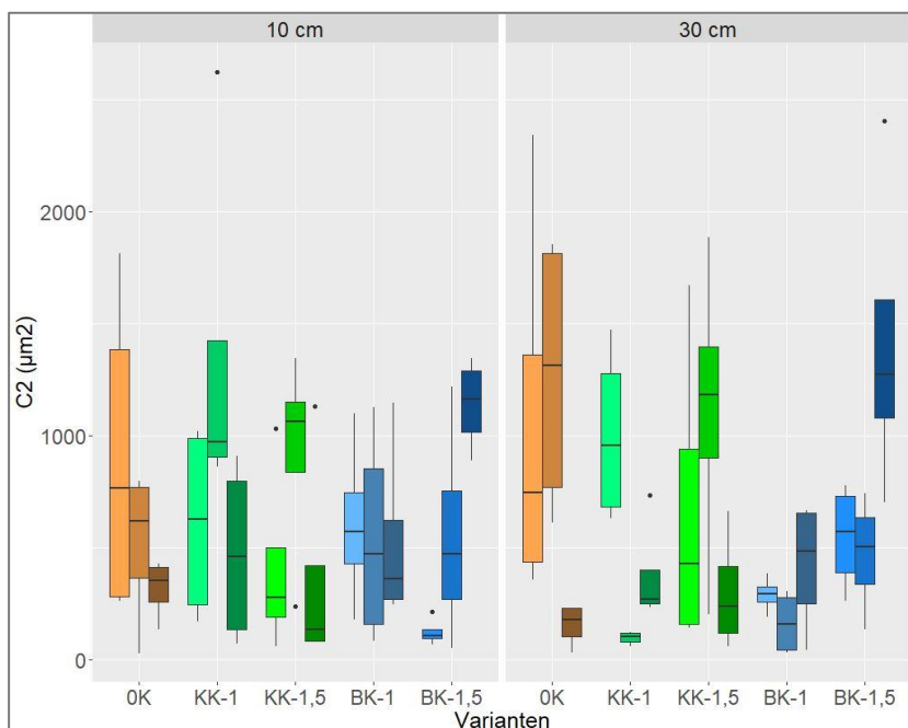
Abbildung 68 C_2 Indices [-], \Psi_m = -60 \text{ hPa} , Standort Struckum, 3 Probenahmen (7, 12 und 26 Monate nach Kalkung). Die drei dunkler werdenden Boxplots einer Farbe symbolisieren die drei Probenahmetermine; n=4 .
