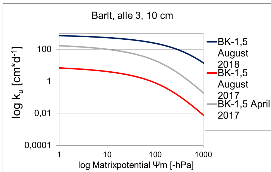
Abbildung 41 Ungesättigte Wasserleitfähigkeit (in \text{cm} \cdot \text{d} ) am Standort Barlt in 10 cm Tiefe für die Variante BK-1,5 für alle 3 Probenahmen 7, 12 und 24 Monate nach Kalkung, n = 4 .
