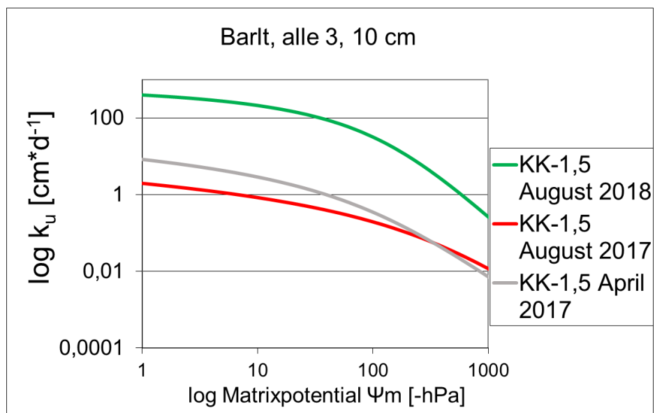
Abbildung 39 Ungesättigte Wasserleitfähigkeit (in \text{cm} \cdot \text{d} ) am Standort Barlt in 10 cm Tiefe für die Variante KK-1,5 für alle 3 Probenahmen 7, 12 und 24 Monate nach Kalkung, n = 4 .
