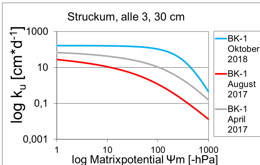
Abbildung 63 Ungesättigte Wasserleitfähigkeit (in \text{cm} \cdot \text{d} ) am Standort Struckum in 30 cm Tiefe für die Variante BK-1 für alle 3 Probenahmen 7, 12 und 26 Monate nach Kalkung, n = 4 .
