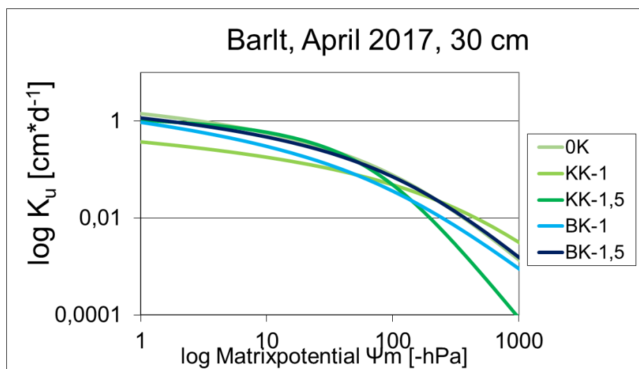
Abbildung 42 Ungesättigte Wasserleitfähigkeit (in \text{cm} \cdot \text{d} ) am Standort Barlt in 30 cm Tiefe, 7 Monate nach Kalkung, n = 4 .
