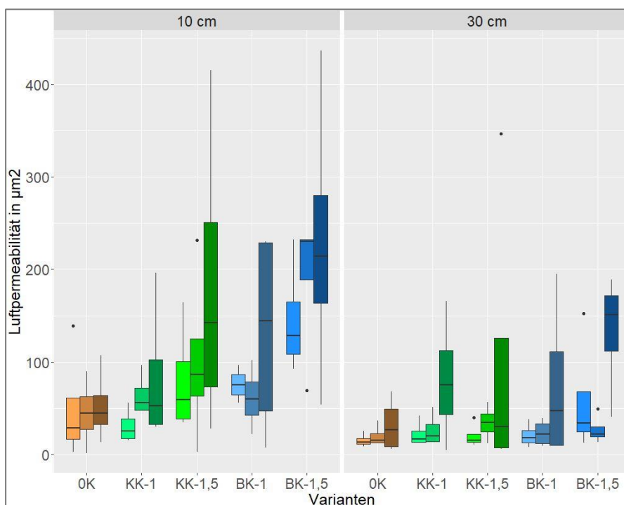
Abbildung 67 Luftpermeabilität (in \mu\text{m}^2 ), \Psi_m = -60 \text{ hPa} , Standort Barlt, 3 Probenahmen (7, 12 und 24 Monate nach Kalkung). Die drei dunkler werdenden Boxplots einer Farbe symbolisieren die drei Probenahmetermine; n=4 .
