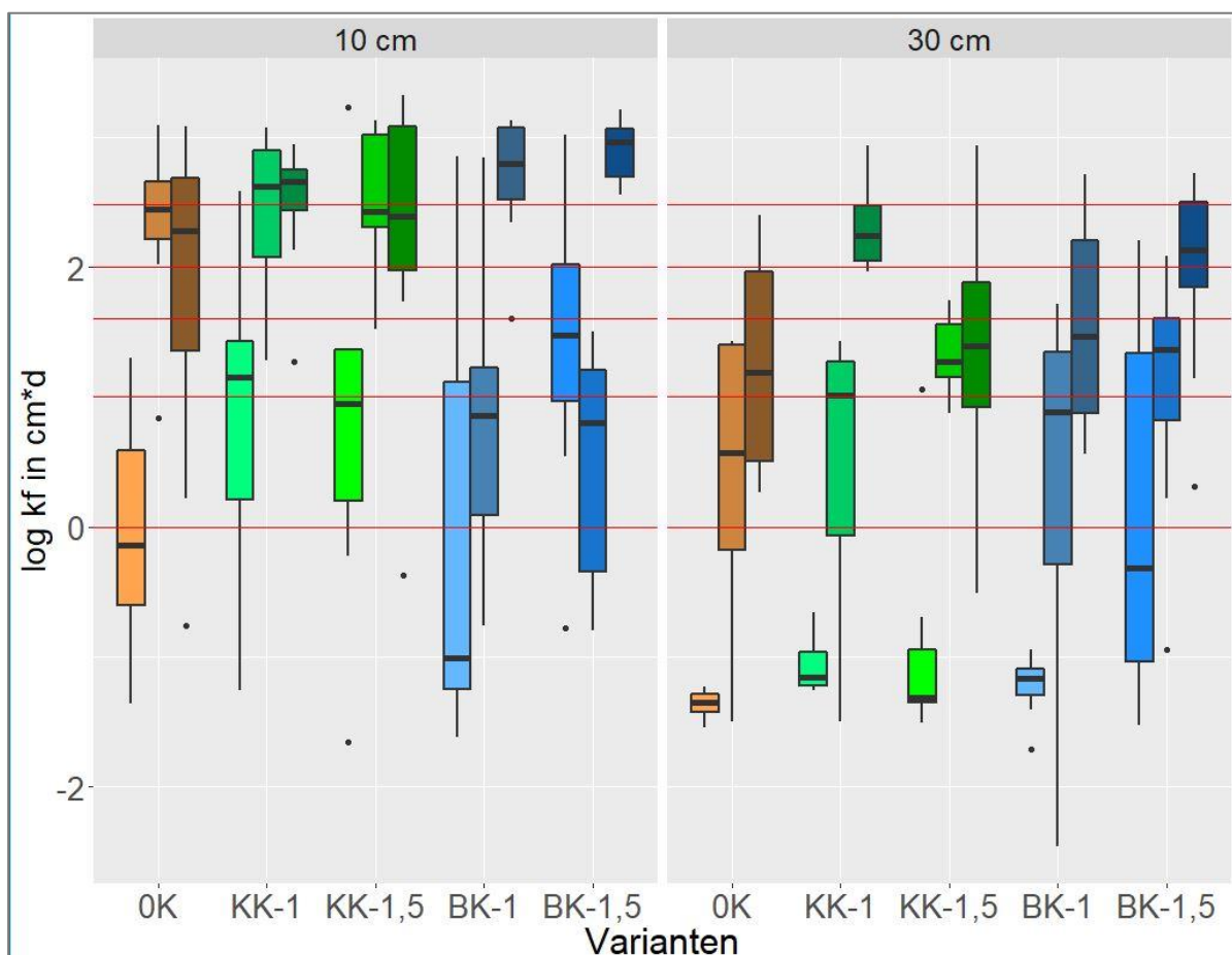
Abbildung 14 Gesättigte Wasserleitfähigkeiten am Standort Barlt in den Tiefen 10 und 30 cm und für drei verschiedene Probenahmeterminen (7, 12 und 24 Monate nach Kalkung), repräsentiert durch die dunkler werdenden Boxplots einer Farbe/Variante. Die roten Linien entsprechen den Grenzwerten der Einstufung nach KA5 (von unten aufsteigend: 1, 10, 40, 100, 300 cm/d). Die Varianten sind: OK = Nullkalk Referenz, KK-1 = Kohlensäurer Kalk in der einfachen Menge nach VDLUFA Empfehlung für den jeweiligen Standort, KK-1,5 = Kohlensäurer Kalk in der anderthalbfachen Menge nach VDLUFA Empfehlung für den jeweiligen Standort, BK-1 = Branntkalk in der einfachen Menge nach VDLUFA Empfehlung für den jeweiligen Standort, BK-1,5 = Branntkalk in der anderthalbfachen Menge nach VDLUFA Empfehlung für den jeweiligen Standort. n = 8
