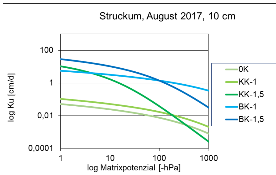
Abbildung 51 Ungesättigte Wasserleitfähigkeit (in \text{cm} \cdot \text{d} ) am Standort Struckum in 10 cm Tiefe, 12 Monate nach Kalkung, n = 4 .
