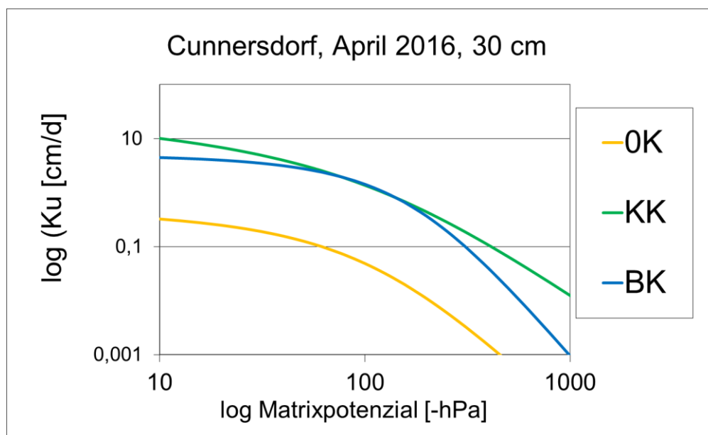
Abbildung 19 Ungesättigte Wasserleitfähigkeit ( k_u in \text{cm} \cdot \text{d} ) für den Standort Cunnersdorf in 30 cm Tiefe, 18 Monate nach letzter Kalkung. Die Varianten sind: OK = Nullkalk Referenz, KK = Kohlensaurer Kalk, BK = Brannkalk.
