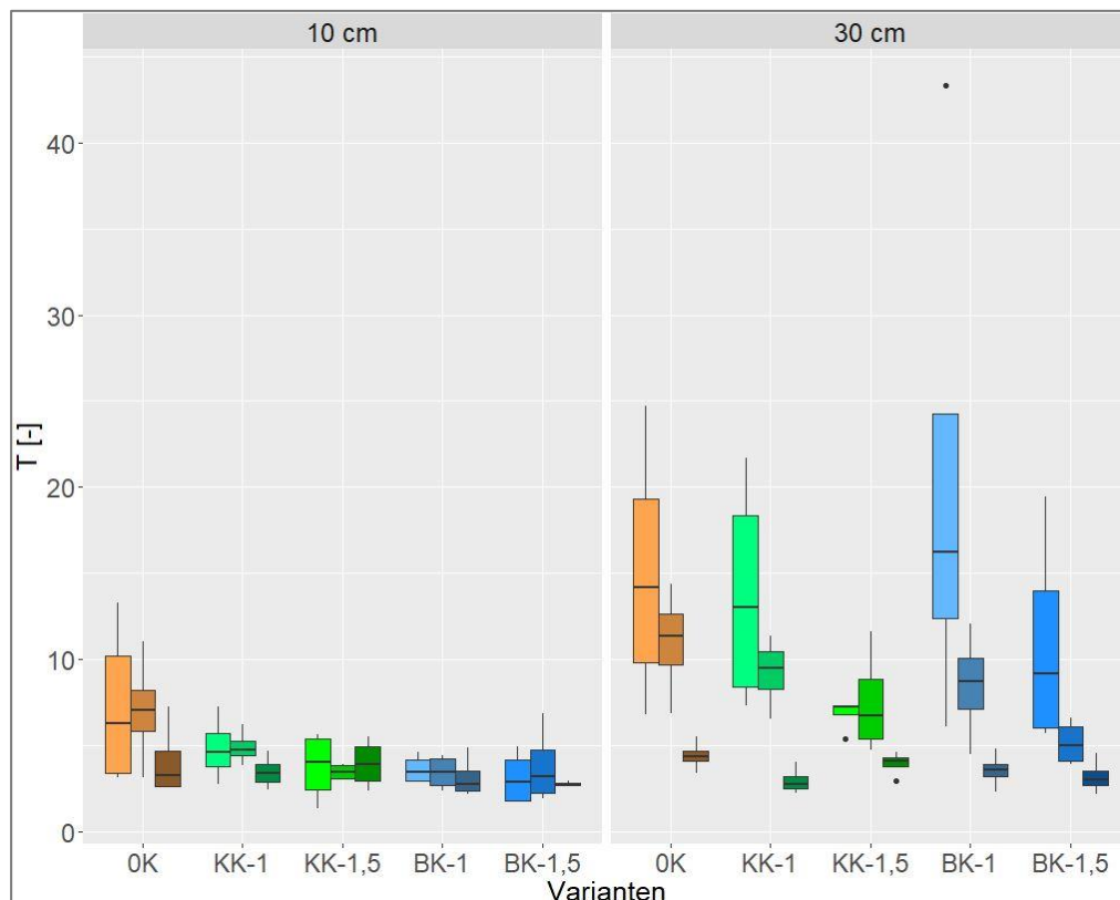
Abbildung 24 Tortuositätsindices ( T [-] ), \Psi_m = -60 hPa, Standort Struckum, 3 Probenahmen (7, 12 und 26 Monate nach Kalkung). Die drei dunkler werdenden Boxplots einer Farbe symbolisieren die drei Probenahmetermine; Die Varianten sind: OK = Nullkalk Referenz, KK-1 = Kohlensaurer Kalk in der einfachen Menge nach VDLUFA Empfehlung für den jeweiligen Standort, KK-1,5 = Kohlensaurer Kalk in der anderthalbfachen Menge nach VDLUFA Empfehlung für den jeweiligen Standort, BK-1 = Branntkalk in der einfachen Menge nach VDLUFA Empfehlung für den jeweiligen Standort, BK-1,5 = Branntkalk in der anderthalbfachen Menge nach VDLUFA Empfehlung für den jeweiligen Standort. n=4 .
