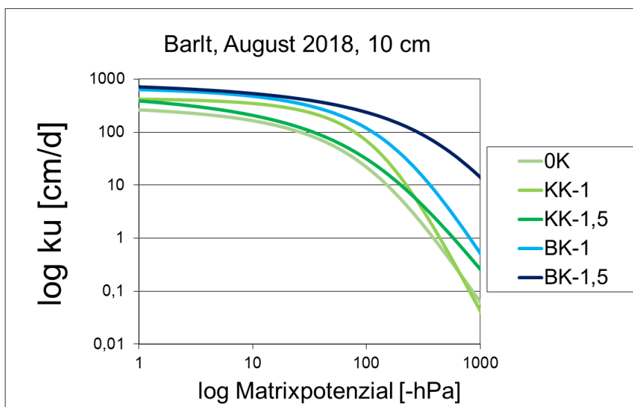
Abbildung 36 Ungesättigte Wasserleitfähigkeit (in \text{cm} \cdot \text{d} ) am Standort Barlt in 10 cm Tiefe, 24 Monate nach Kalkung, n = 4 .
