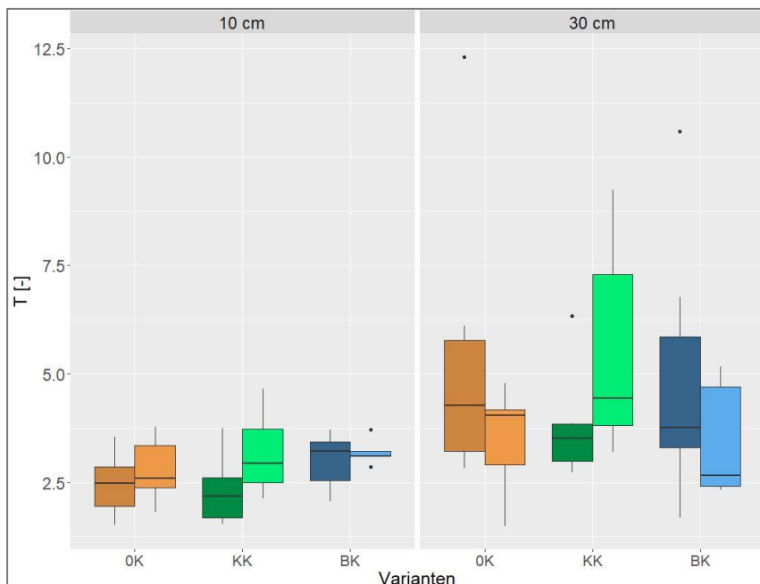
Abbildung 71 Tortuositätsindices T [-] , \Psi_m = -60 hPa, Standort Cunnersdorf an 2 Probenahmen 18 (linker Boxplot) und 23 Monate (rechter Boxplot) nach letzter Kalkung, n = 4 .
