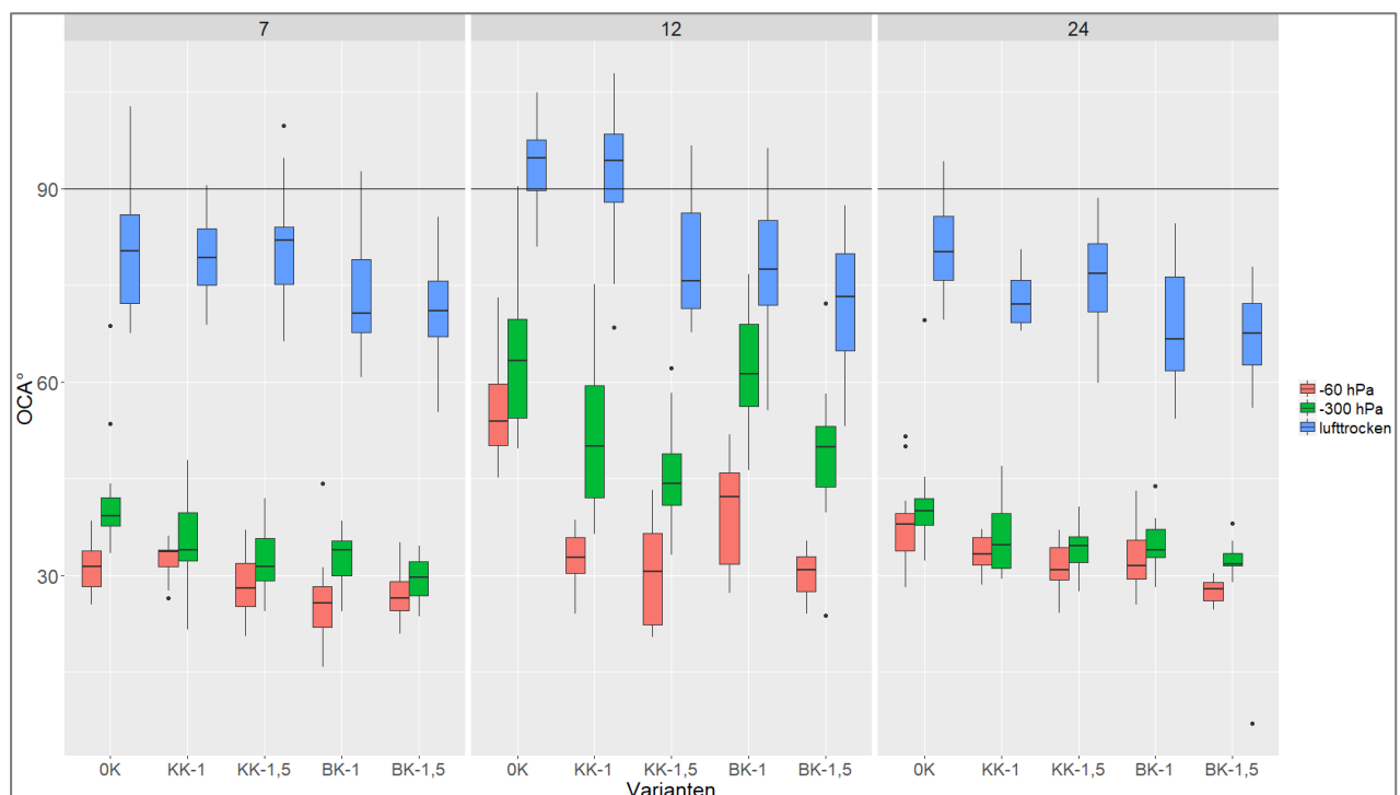
Abbildung 30 Optische Kontaktwinkel am Standort Barlt in 10 cm Tiefe für die drei Probenahmeterminen 7, 12 und 24 Monate nach Kalkung, gemessen an 3 unterschiedlichen Entwässerungsstadien (-60 hPa in Rot, -300 hPa in Grün und lufttrocken in Blau).. Die schwarze horizontale Linie verläuft bei 90°, oberhalb dessen die Werte als benetzungshemmend gelten (Bachmann et al., 2013). Die Varianten sind: OK = Nullkalk Referenz, KK-1 = Kohlensaurer Kalk in der einfachen Menge nach VDLUFA Empfehlung für den jeweiligen Standort, KK-1,5 = Kohlensaurer Kalk in der anderthalbfachen Menge nach VDLUFA Empfehlung für den jeweiligen Standort, BK-1 = Brantkalk in der einfachen Menge nach VDLUFA Empfehlung für den jeweiligen Standort, BK-1,5 = Brantkalk in der anderthalbfachen Menge nach VDLUFA Empfehlung für den jeweiligen Standort. n = 16
