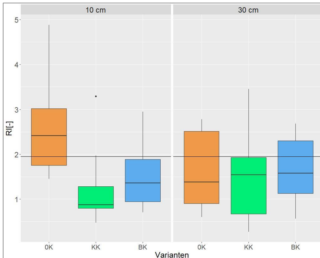
Abbildung 29 Repellency Indices am Standort Cunnersdorf (RI, dimensionslos, gemessen bei \Psi_m = -60 hPa) für die Tiefen 10 und 30 cm, 23 Monate nach letzter Kalkung. Die schwarze horizontale Linie verläuft bei einem Wert von 1,95 der nach einigen Literaturquellen als kritischer Grenzwert fungiert, oberhalb dessen Benetzungshemmung auftritt. Die Varianten sind: OK = Nullkalk Referenz, KK = Kohlensäurer Kalk, BK = Branntkalk. n = 12
